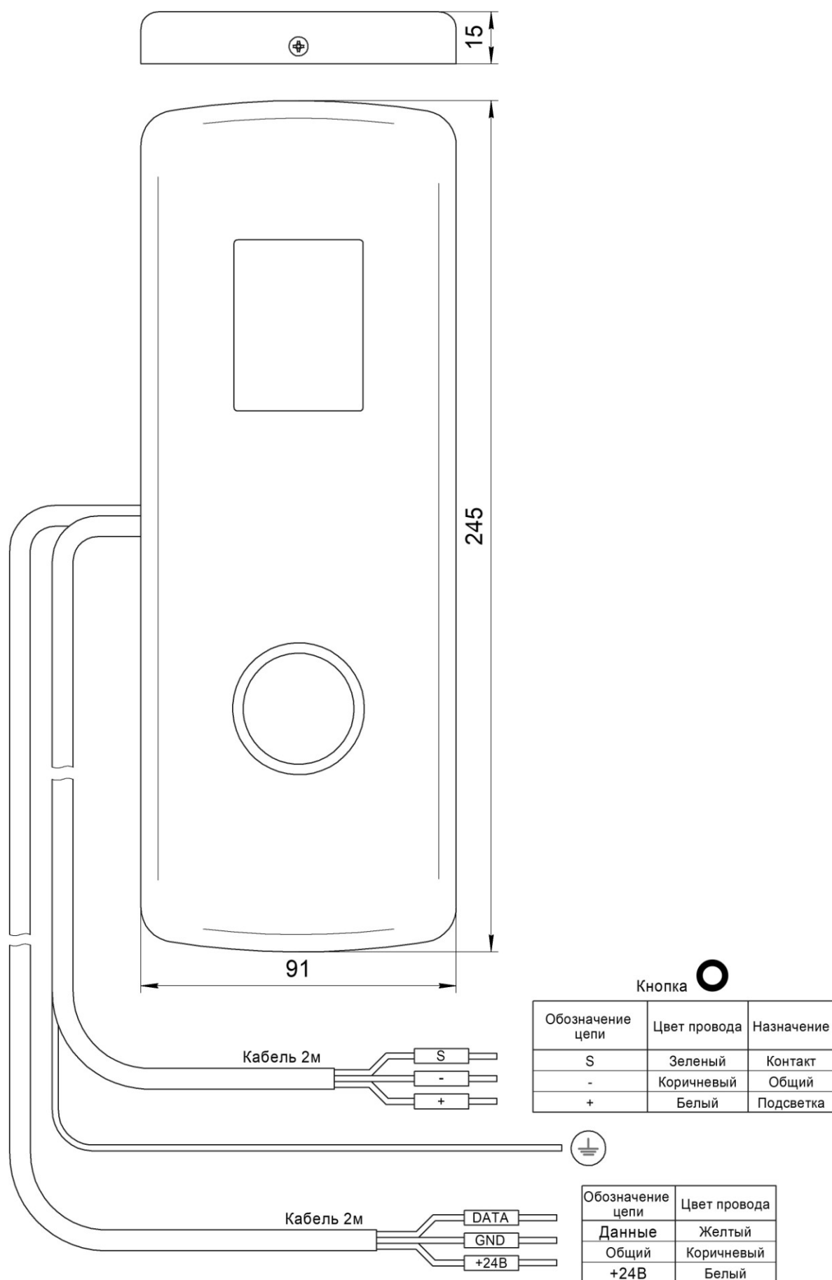
Рис.1 Внешний вид, габаритные и установочные размеры Вызывного поста ЦИРКОН НШЕК.468381.029
